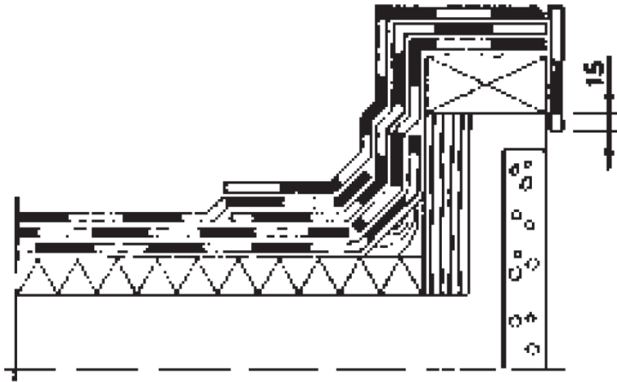
Bild 6. Takskägg, tredubbelt tätskikt.
