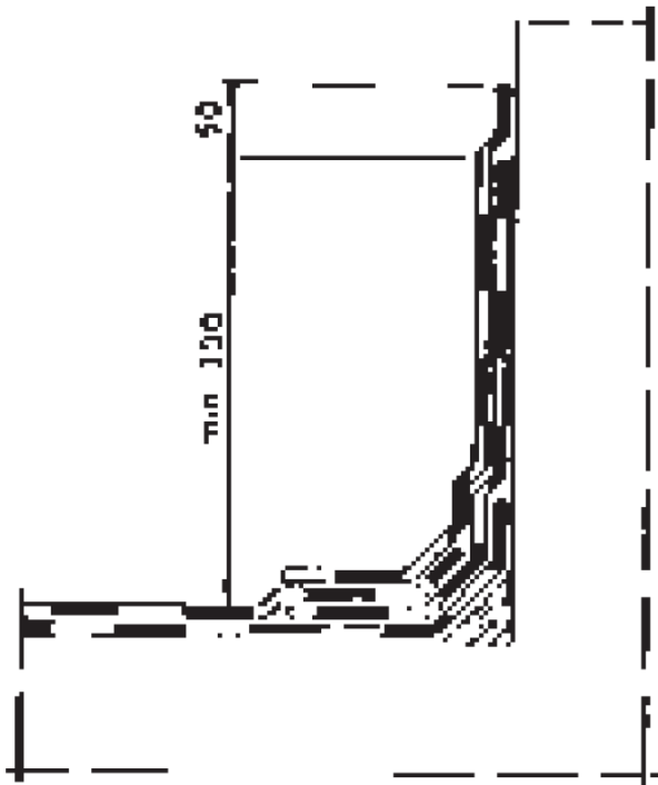
Bild 8. Upp mot vägg, dubbelt tätskikt.
