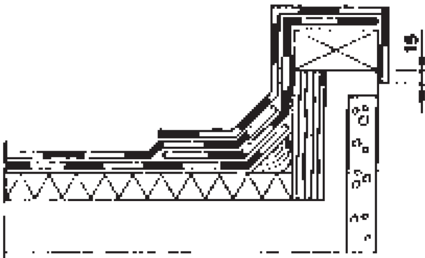
Bild 5. Takskägg, dubbelt tätskikt.
