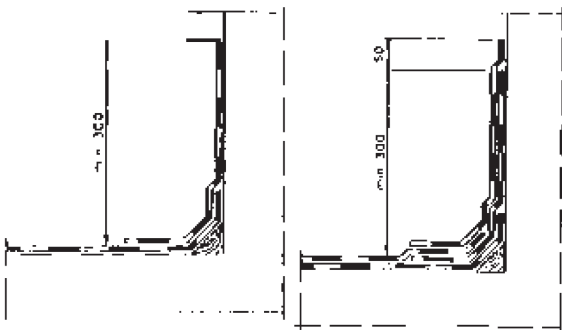
Bild 7. Upp mot vägg, enkelt tätskikt.
