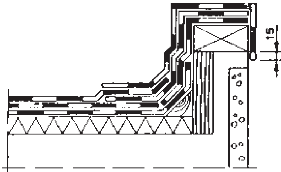
Bild 6. Takskägg, tredubbelt tätskikt.
