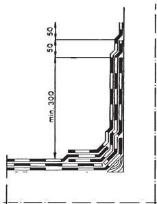
Kuva 9. Seinällennosto, 3-kermikate.
