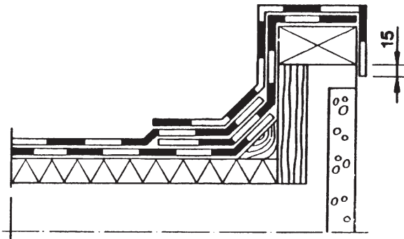
Kuva 5. Räystäs, 2-kermikate.
