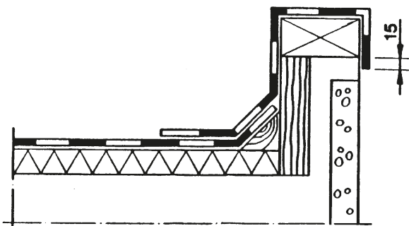
Kuva 4. Räystääs, 1-kermikate.
