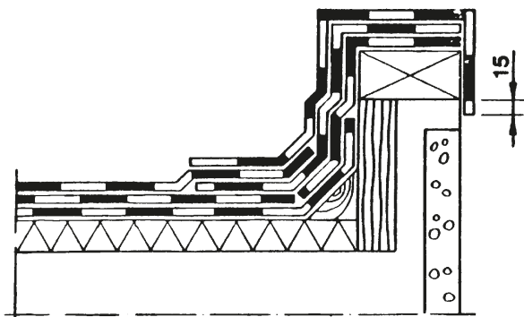
Kuva 6. Rästäs, 3-kermikate.
