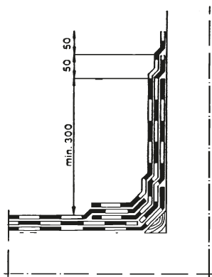
Kuva 9. Seinällennosto, 3-kermikate.
