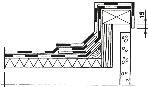
Kuva 5. Räystääs, 2-kermikate.
