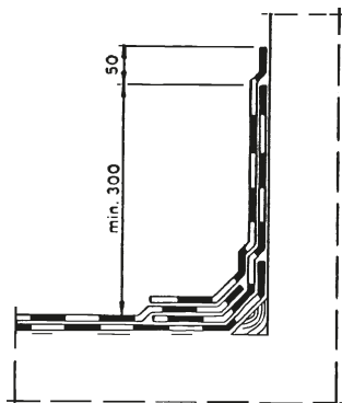
Kuva 8. Seinällenosto, 2-kermikate.
