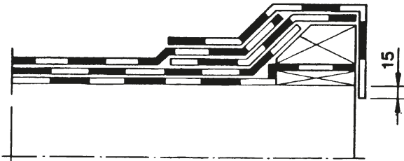
Kuva 2. Saneeraustyö, korotettu räystäs, 2-kermikate.
