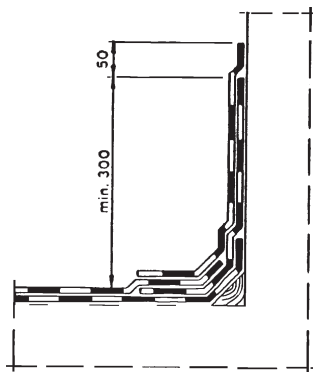
Kuva 8. Seinälienenosto, 2-kermikate.
