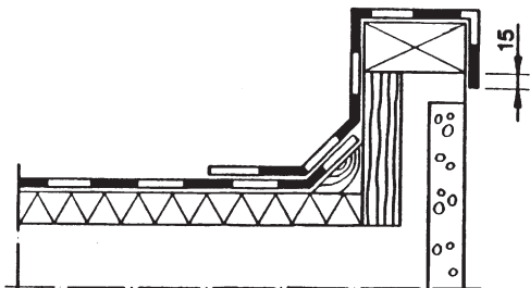
Kuva 4. Räystäs, 1-kermikate.
