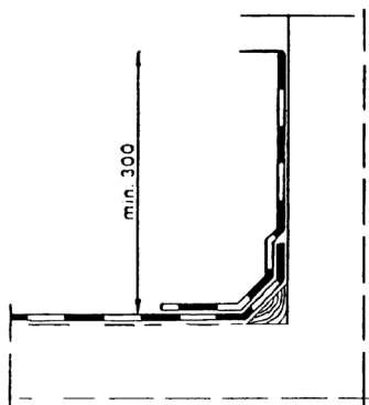
Bild 7. Upp mot vägg, enkelt tätskikt.
