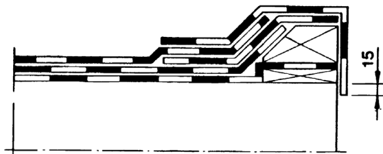
Bild 2. Saneringsarbete, takskägg med upphöjd kant, dubbelt tätskikt.
