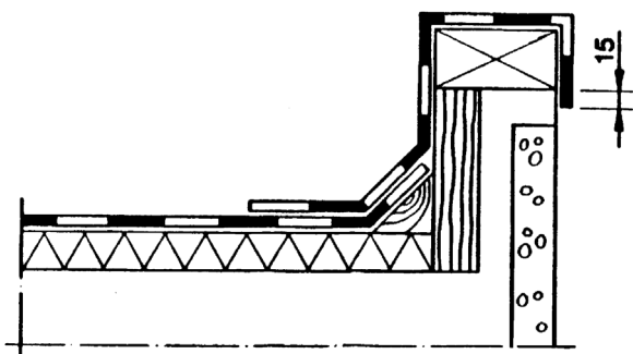
Bild 4. Takskägg, enkelt tätskikt.
