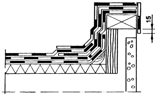
Bild 6. Takskägg, tredubbelt tätskikt.
