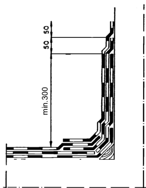
Bild 9. Upp mot vägg, tredubbelt tätskikt.
