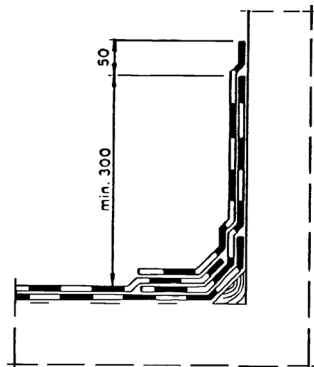
Bild 8. Upp mot vägg, dubbelt tätskikt.
