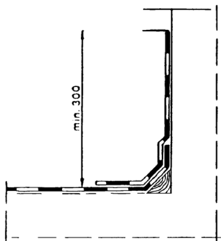
Bild 7. Upp mot vägg, enkelt tätskikt.
