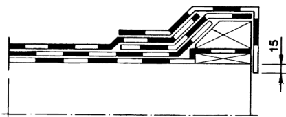
Bild 2. Saneringsarbete, takskägg med upphöjd kant, dubbelt tätskikt.
