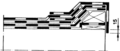
Bild 3. Saneringsarbete, upphöjd kant, tredubbelt tätskikt.
