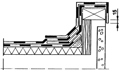
Bild 5. Takskägg, dubbelt tätskikt.
