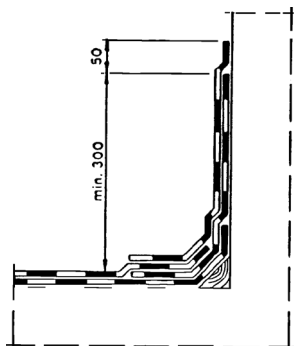
Bild 8. Upp mot vägg, dubbelt tätskikt.
