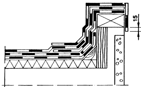
Bild 6. Talskäg, tredubbelt tätskikt.
