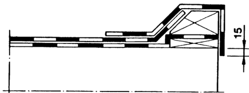
Bild 1. Saneringsarbete, takskägg med upphöjd kant, enkelt tättskikt.
