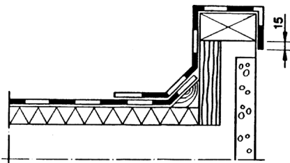
Bild 4. Takskägg, enkelt tätskikt.
