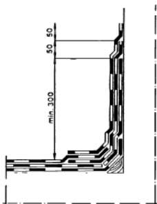
Bild 9. Upp mot vägg, tredubbelt tätskikt.
