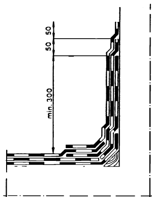
Kuva 9. Seinällenosto, 3-kermikate.
