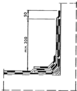
Kuva 8. Seinälienenosto, 2-kermikate.
