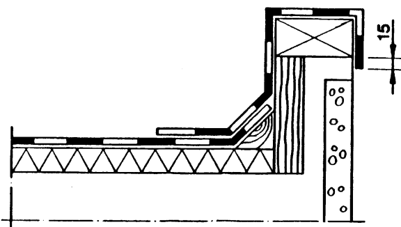
Kuva 4. Räystäs, 1-kermikate.
